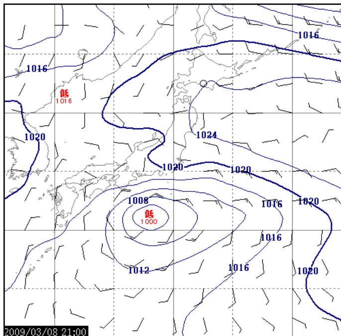
2009/03/08 21:00 T=96 等値線: 気圧(4hPa) 矢羽: 風向・風速(m/s)
