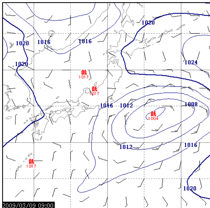
2009/03/09 09:00 T=108 等値線: 気圧(4hPa) 矢羽: 風向・風速(m/s)
