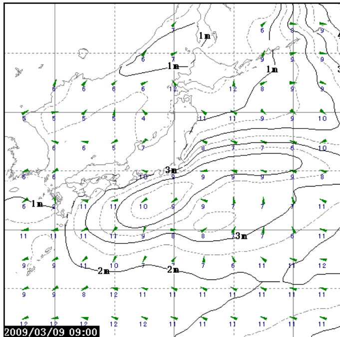
2009/03/09 09:00 T=108 等値線: 波高(0.5m) 矢じり: 波向 数値: 周期(s)
