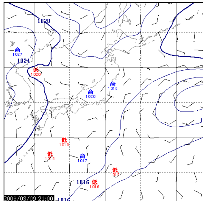
2009/03/09 21:00 T=120 等値線: 気圧(4hPa) 矢羽: 風向・風速(m/s)
