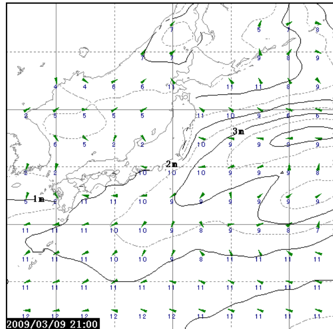
2009/03/09 21:00 T=120 等値線: 波高(0.5m) 矢じり: 波向 数値: 周期(s)
