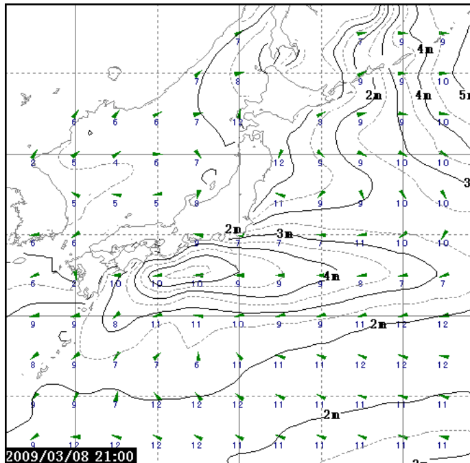
2009/03/08 21:00 T=96 等値線: 波高(0.5m) 矢じり: 波向 数値: 周期(s)
