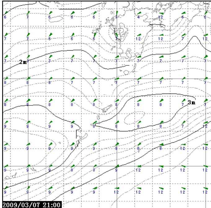
2009/03/07 21:00 T=72 等値線: 波高(0.2m) 矢じり: 波向 数値: 周期(s)
