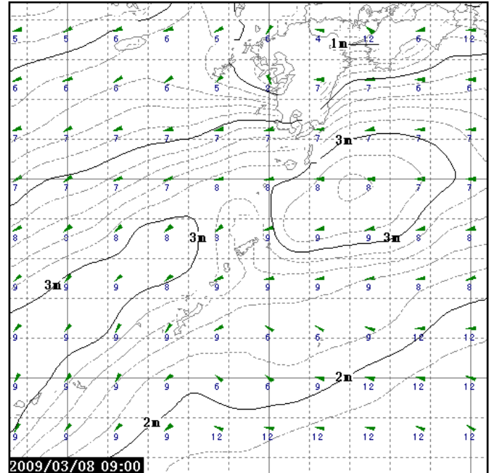
2009/03/08 09:00 T=84 等値線: 波高(0.2m) 矢じり: 波向 数値: 周期(s)
