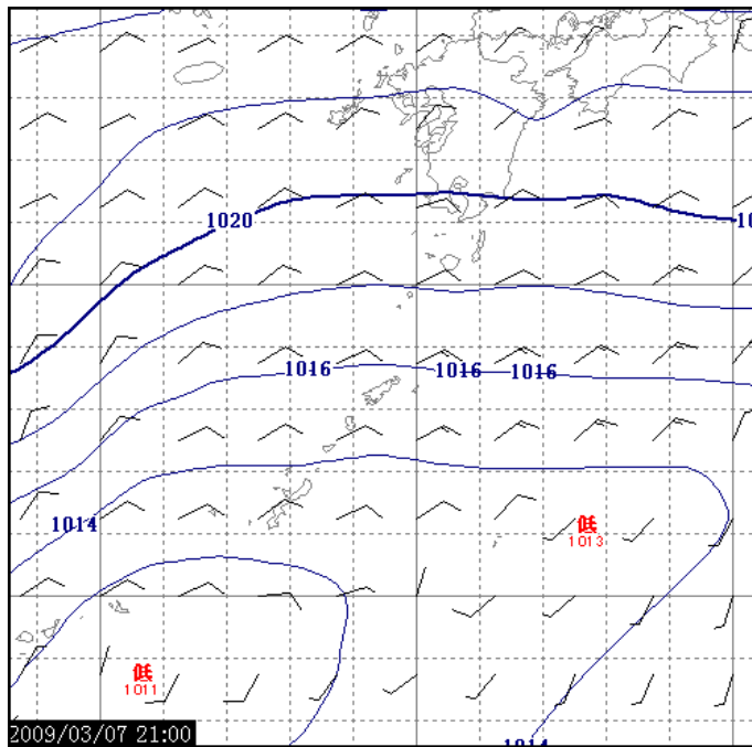
2009/03/07 21:00 T=72 等値線: 気圧(2hPa) 矢羽: 風向・風速(m/s)
