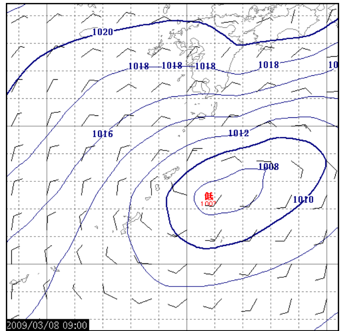
2009/03/08 09:00 T=84 等値線: 気圧(2hPa) 矢羽: 風向・風速(m/s)
