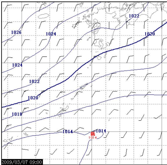
2009/03/07 09:00 T=60 等値線: 気圧(2hPa) 矢羽: 風向・風速(m/s)
