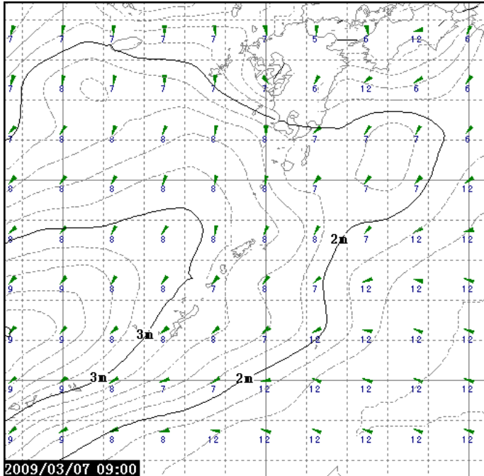
2009/03/07 09:00 T=60 等値線: 波高(0.2m) 矢じり: 波向 数値: 周期(s)
