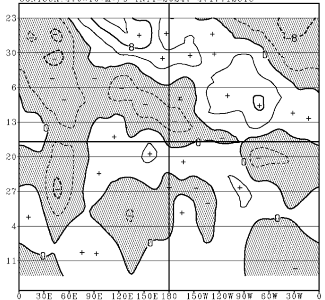
200hPa速度ポテンシャル偏差 (5N-5S) アンサンブル平均 CONTOUR: 4.0 \times 10^6 \text{ m}^2/\text{s} INIT=2024. 4.17.12UTC
